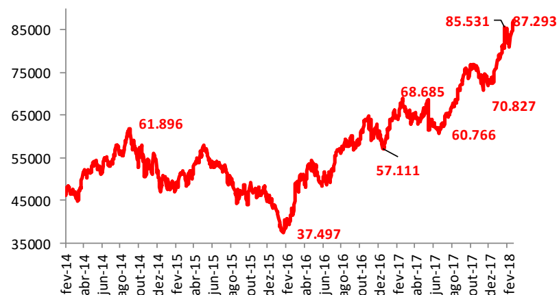
Ibovespa Diário - Fechamento
