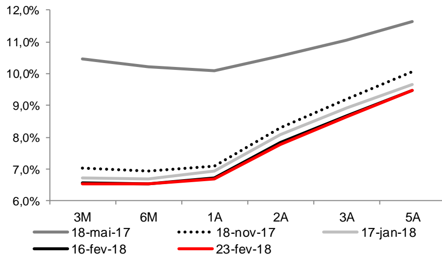
Curva de juros - Brasil
